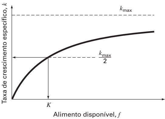
FIGURA 20.1 Gráfico da taxa de crescimento específico em função do alimento disponível para o modelo de taxa de crescimento saturado usado para caracterizar a cinética microbial. O valor K é chamado de constante de meia saturação porque corresponde à concentração na qual a taxa de crescimento específico é a metade de seu valor máximo.
