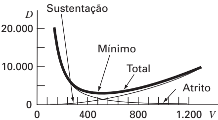
Figura P16.27 Gráfico do arrasto versus a velocidade para um aerofólio.
