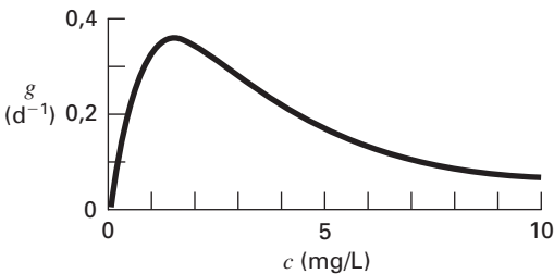
Figura P16.3 Taxa de crescimento específico de uma cultura que produz antibiótico versus a concentração de alimento.
