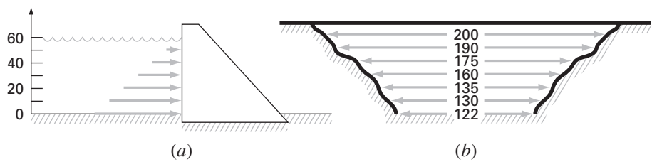
Figura P24.22 Água exercendo pressão na face a montante de um dique: (a) visão lateral mostrando a força linearmente crescente com a profundidade; (b) visão frontal mostrando a largura da represa em metros.
